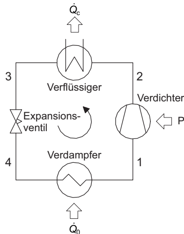
Abb. 1.43: Schema einer einstufigen Kälteanlage
