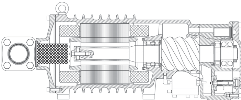
Abb. 2.10: Integrierte Leistungsregelung eines Schraubenverdichters (Bitzer)
