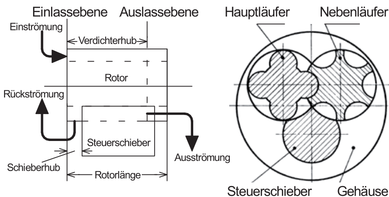
Abb. 2.11: Schema der Fördermengenregelung mit einem Steuerschieber (MAN/GHH)
