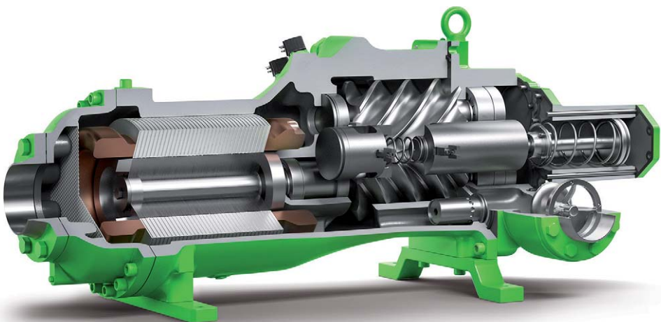
Abb. 2.9: Schnitt durch einen halbhermetischen Schraubenverdichter (Bitzer)
