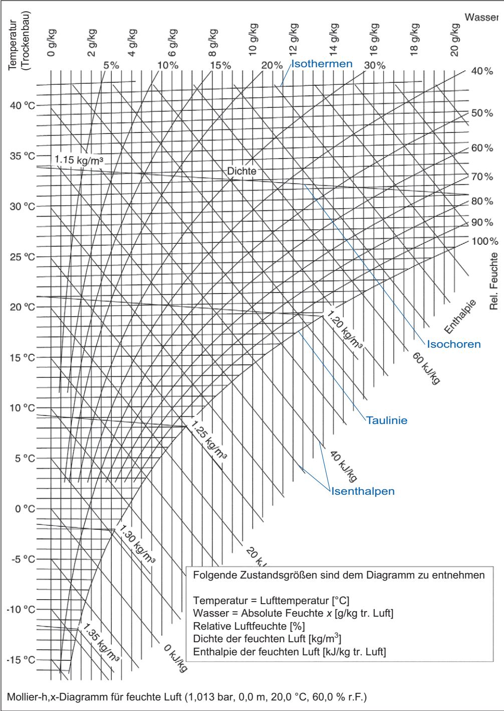
Abb. 1.35: Mollier-h,x-Diagramm für feuchte Luft
