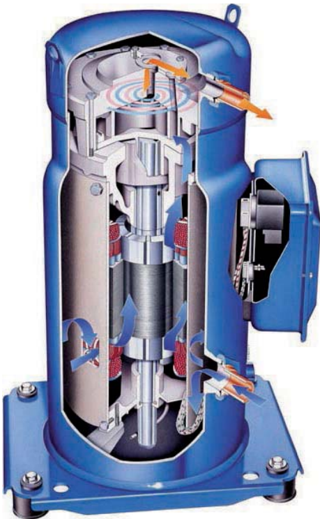
Abb. 2.7: Scrollverdichter (Danfoss)
