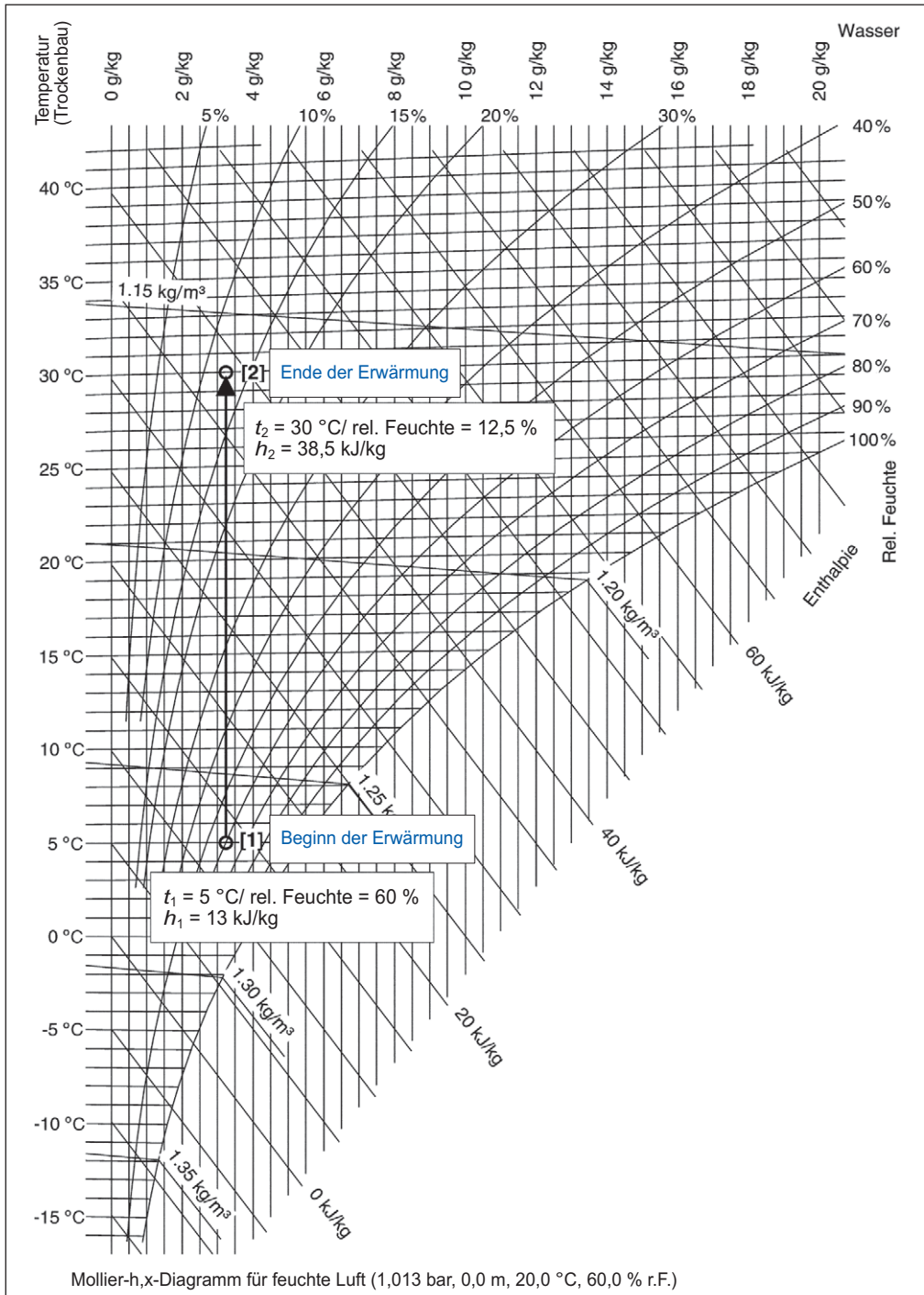
Abb. 1.36: Erwärmung
