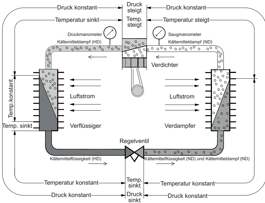
Abb. 1.42: Schema Kältemittelkreislauf mit stetig regelndem Ventil als Drosselorgan
