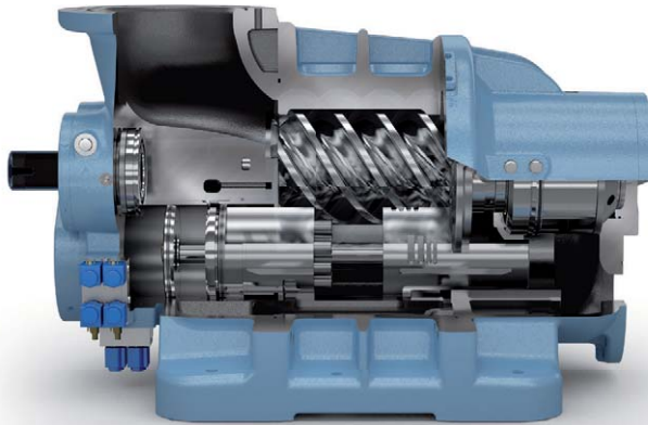
Abb. 2.12: Schnitt durch einen Schraubenverdichter, mit Leistungsregelung und verstellbarem VI (GEA Refrigeration Germany)
